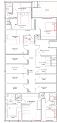
PLANTA SÓTANO, DESPUÉS DE LIFO
