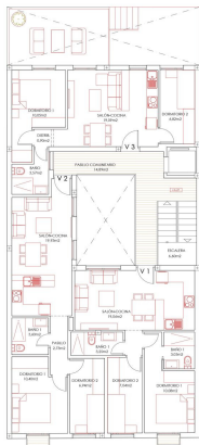
PLANTA SEGUNDA
